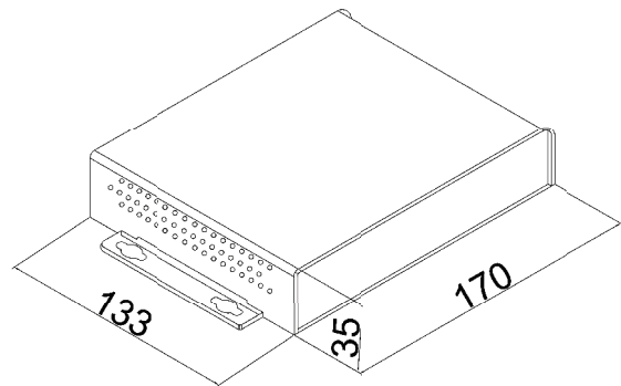
整体尺寸 (单位: mm)
